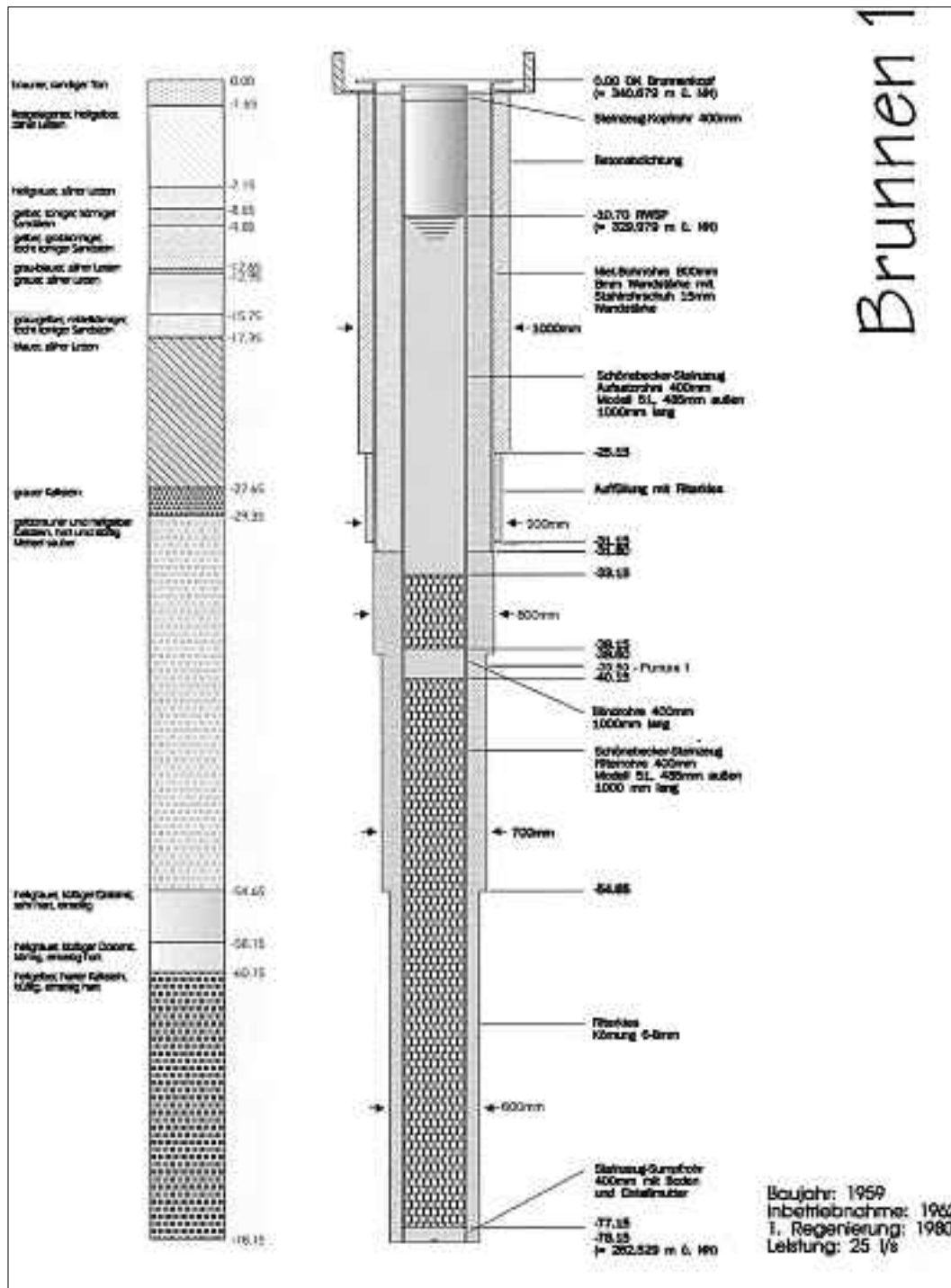
Die Grafik zeigt links die Erd- und Gesteinsschichten und rechts die für die Förderung notwendige technische Ausrüstung.
